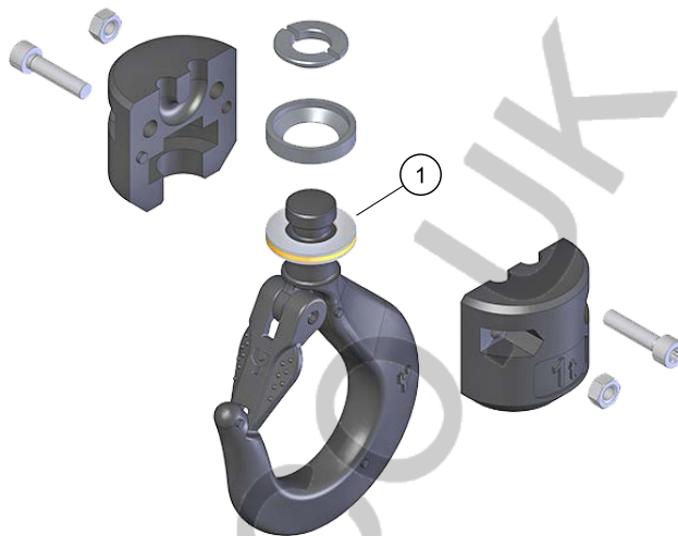
1 Rolamento axial
