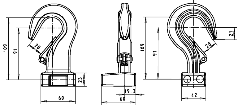
EUROCHAIN VL2 & 5
